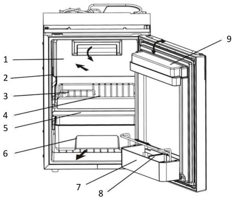
Рис.1 MC-CRX-50
