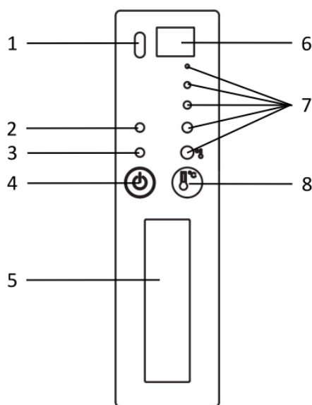
Рис.3 Панель управления
