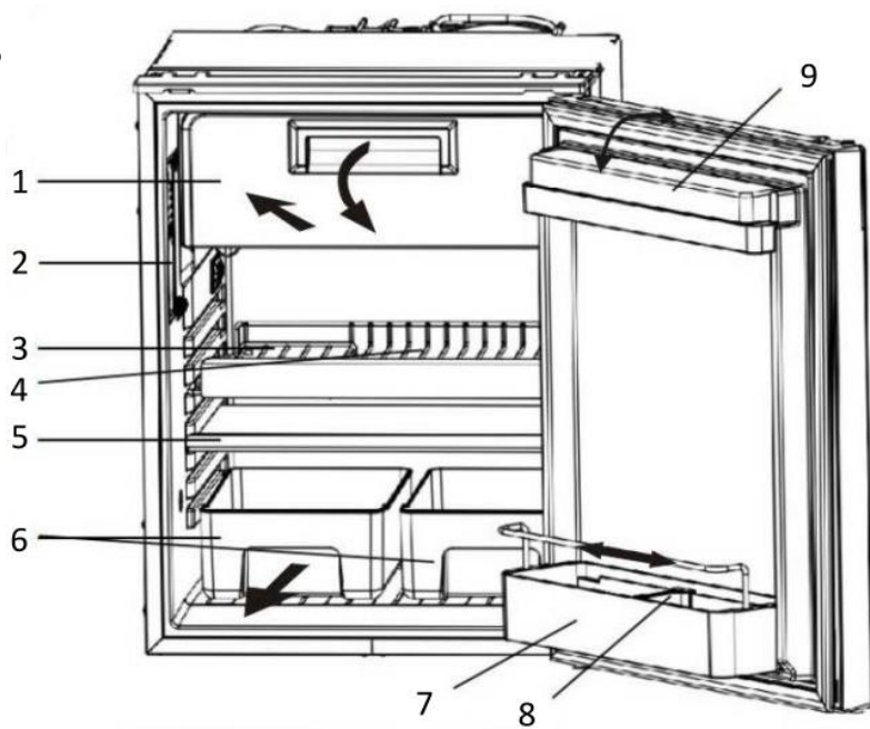
Рис.2 MC-CRX-85
